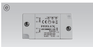
e Dimming Interface (1-10V) : FDC-L10
